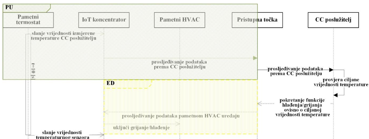
Slika 3.5 UML dijagram međudjelovanja komunikacijskog procesa u kojemu se generiraju PU i ED uzorci prometa
