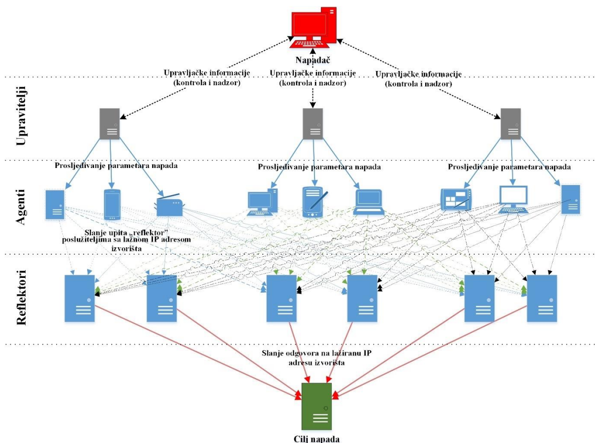
Slika 4.7 Izvođenje DDoS napada posredstvom "reflektor" poslužitelja
