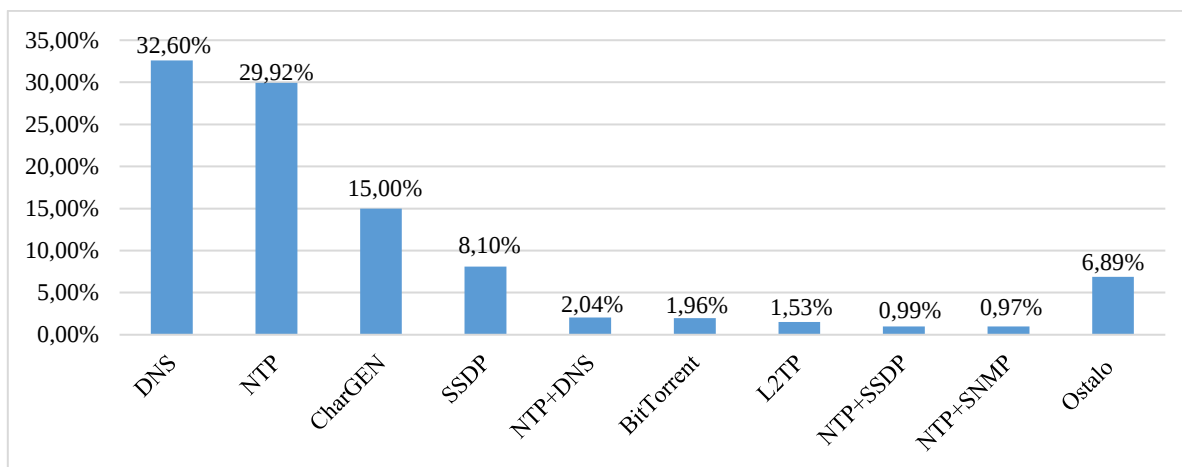
Grafikon 4.4 Protokoli korišteni u DRDoS napadima
