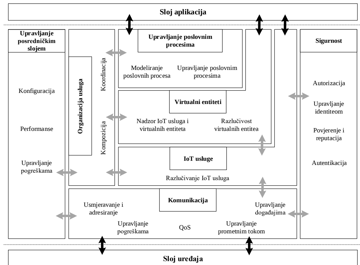
Slika 2.3 Arhitektura posredničkog sloja koncepta IoT [77]
