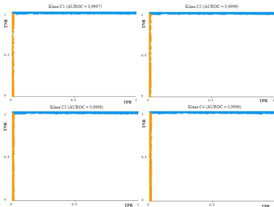
Slika 5.9 Prikaz ROC krivulje za klasifikacijski model M4
