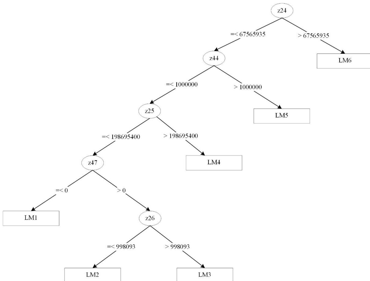
Slika 5.12 Prikaz LMT modela detekcije anomalija mrežnoga prometa za klasu C4
