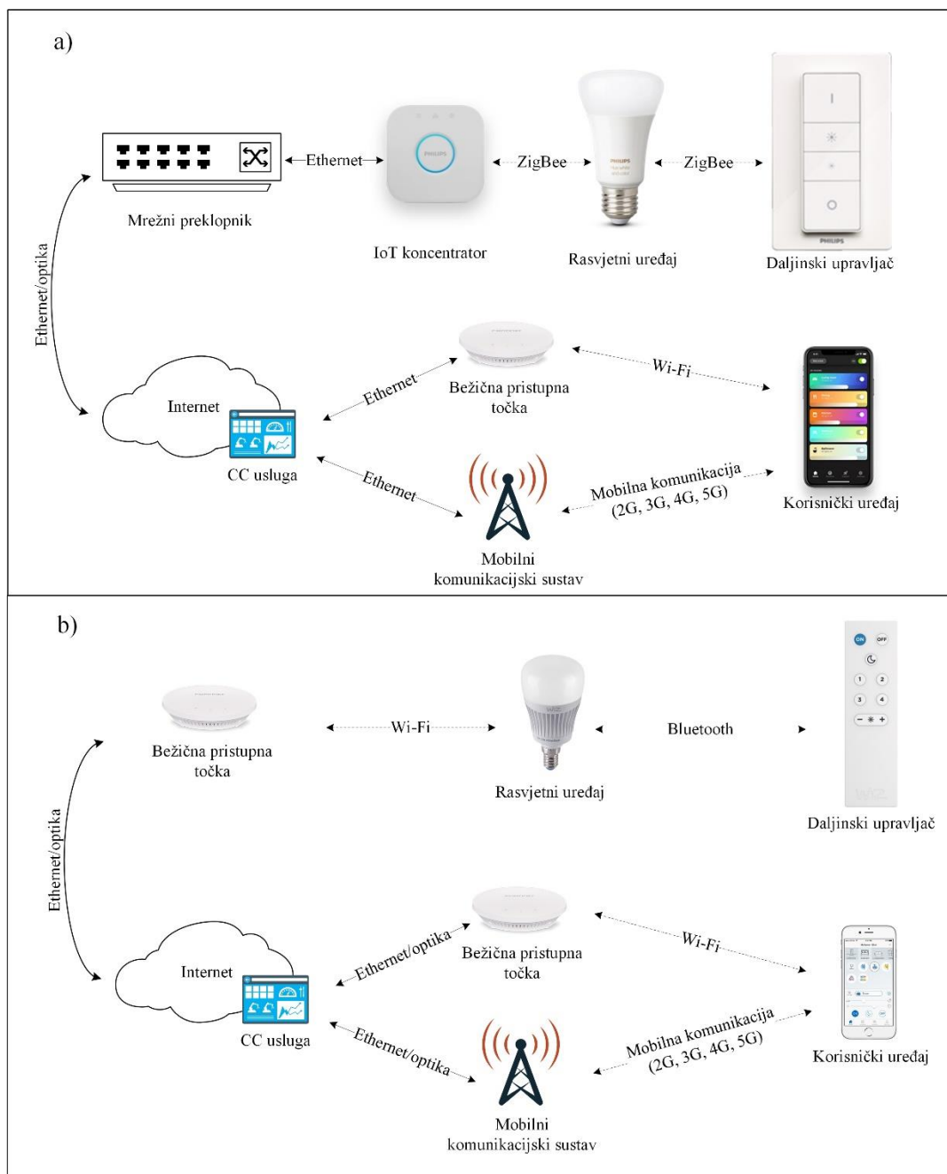
Slika 3.3 Scenariji povezivanja SHIoT uređaja u okruženju pametnog doma; a) uz IoT konzentator i žičanu komunikaciju i b) bez IoT konzentatora i isključivo bežičnom komunikacijom
